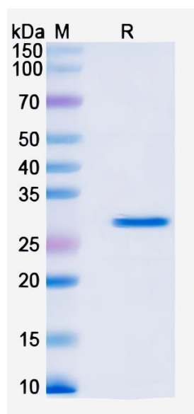
SDS-PAGE
