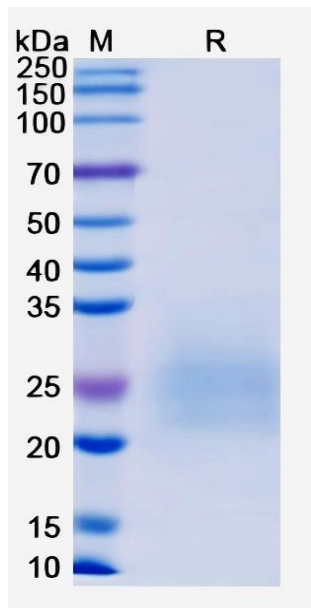
SDS-PAGE
