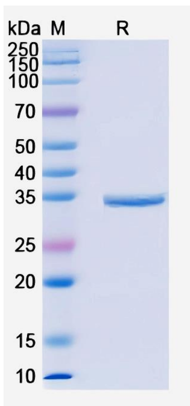
SDS-PAGE
