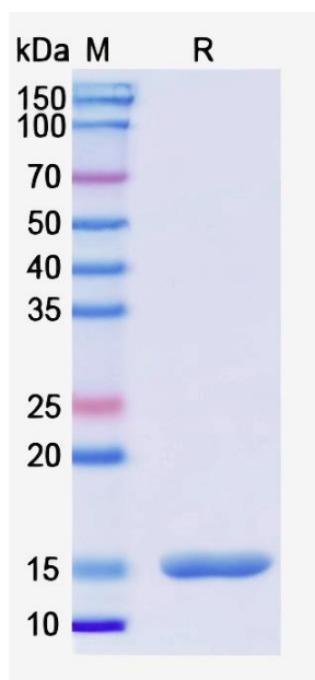
SDS-PAGE
