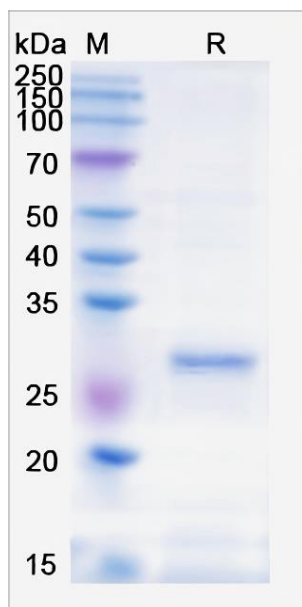
SDS-PAGE
