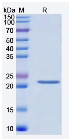
SDS-PAGE
