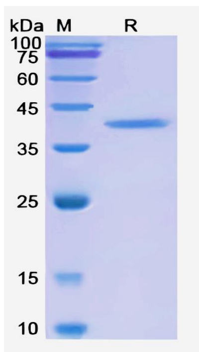
SDS-PAGE
