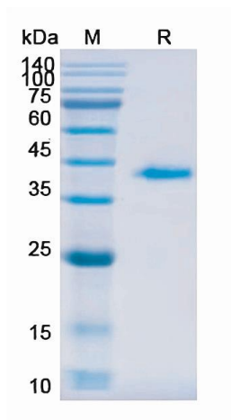
SDS-PAGE
