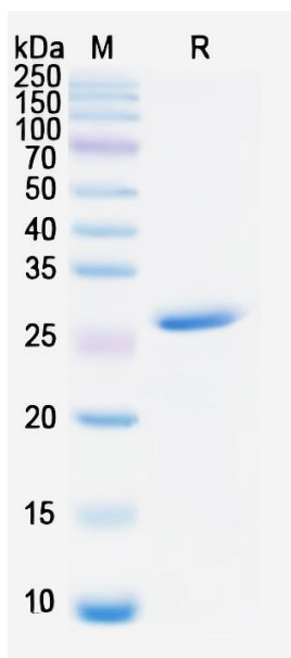
SDS-PAGE
