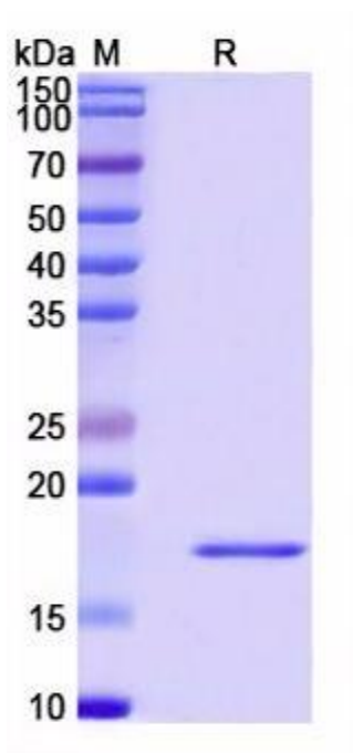
SDS-PAGE
