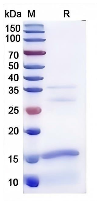
SDS-PAGE
