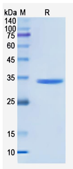
SDS-PAGE
