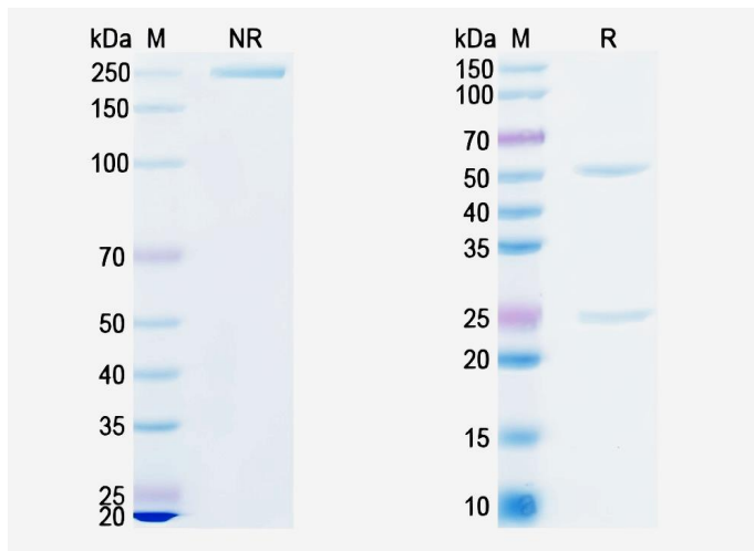
SDS-PAGE
