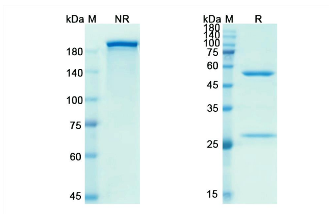
SDS-PAGE
