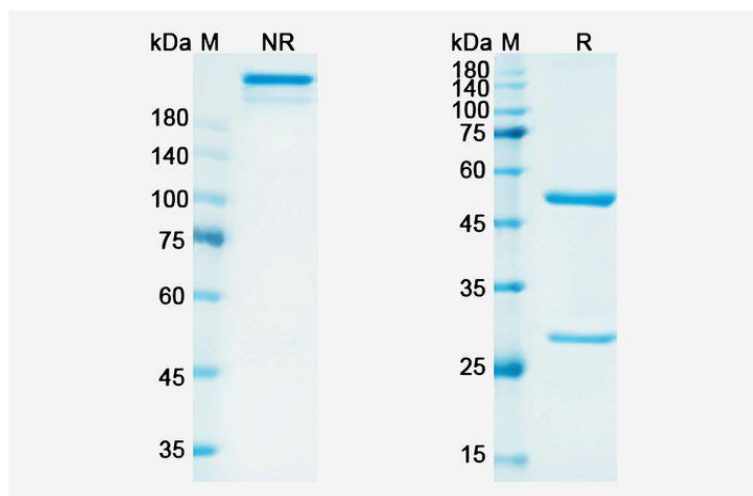
SDS-PAGE
